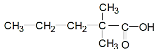
2,2-diméthylpentanoïque
